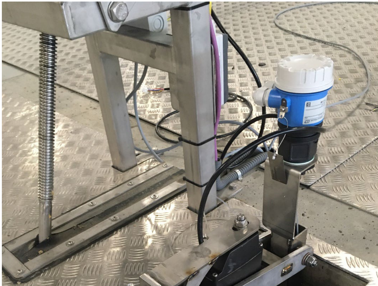
VE-Designet flowmåler på indløb til procestanke.
